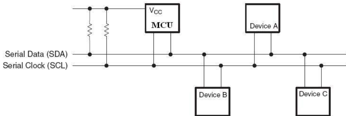
I 2 C 总线连线图
